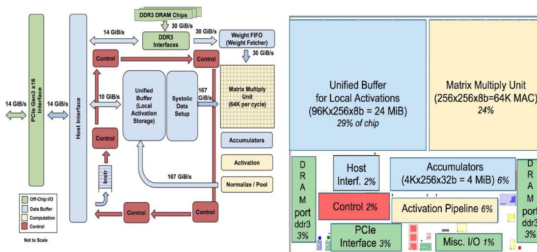
Рис. 3. Архитектура тензорного процессора TPU v1.
