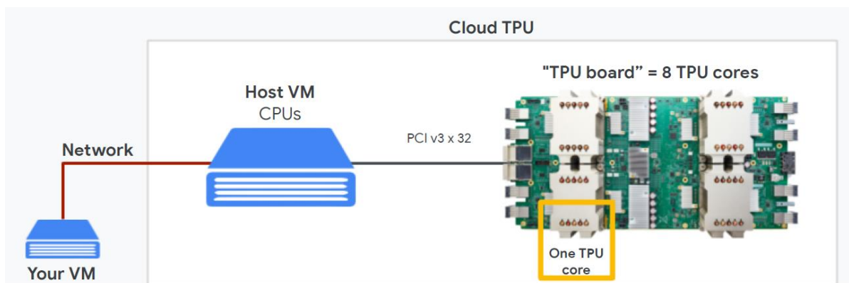
Рис. 4. Организация управления TPU в облаке.
