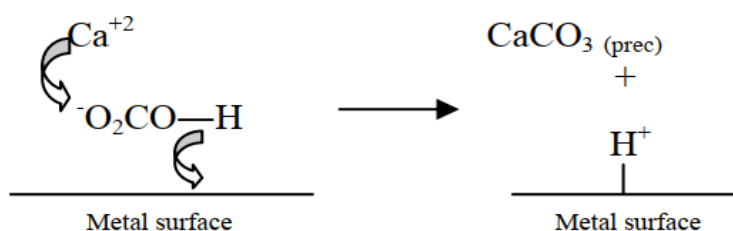
Рис. 3. Схема реакции образования карбоната кальция и водорода
