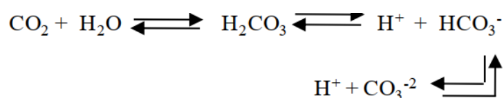
Рис. 1. Схема реакций образования угольной кислоты
