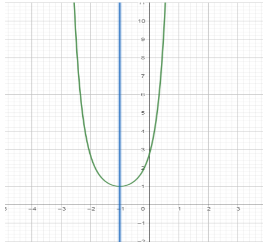
Рис. 1. График функции f(x) = e^{x^2+2x+1}
