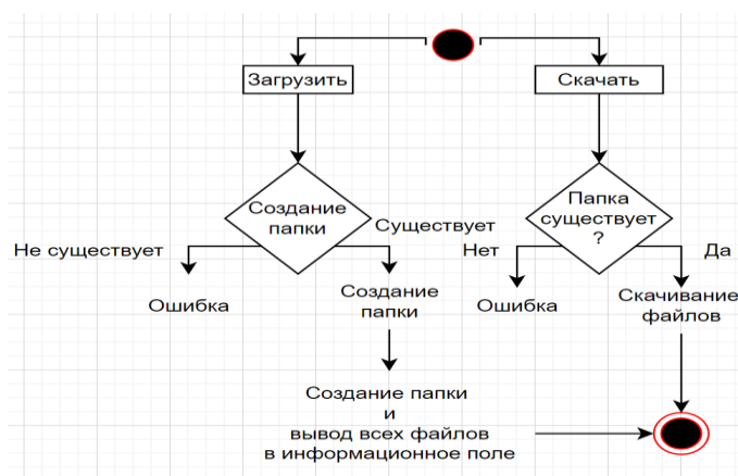
Рис. 2. Алгоритм взаимодействия с облачным хранилищем данных
