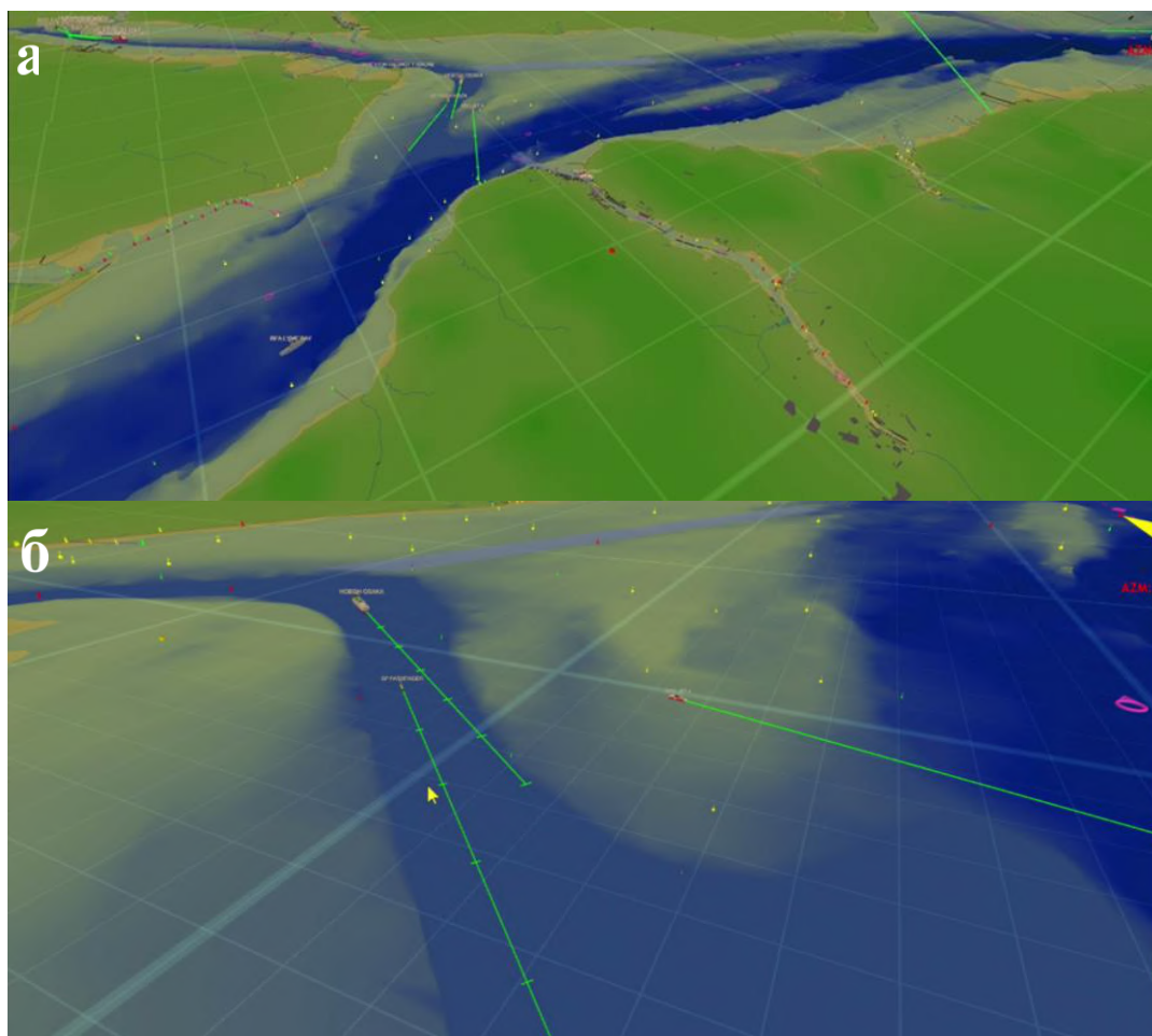
Рис. 2. Примеры представления информации о подходных путях порта Саутгемптон по 3D ЭНК различного масштаба: а) мелкого; б) крупного
