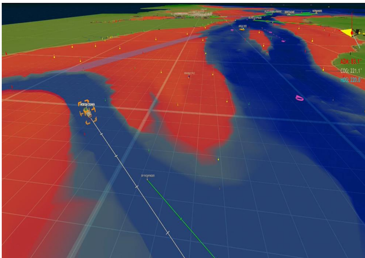
Рис. 3. Фрагмент 3D ЭНК, отображающий область опасных глубин, на сложном в навигационном отношении участке подходного фарватера порта
