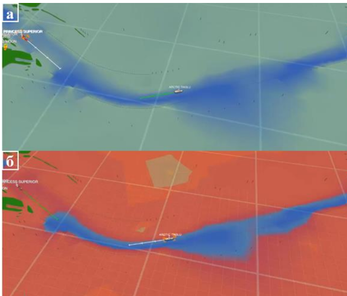
Рис. 4. Представление информации о глубинах на 3D ЭНК: а) без учета осадки судна; б) в виде области опасных и безопасных глубин применительно к осадке выбранного судна
