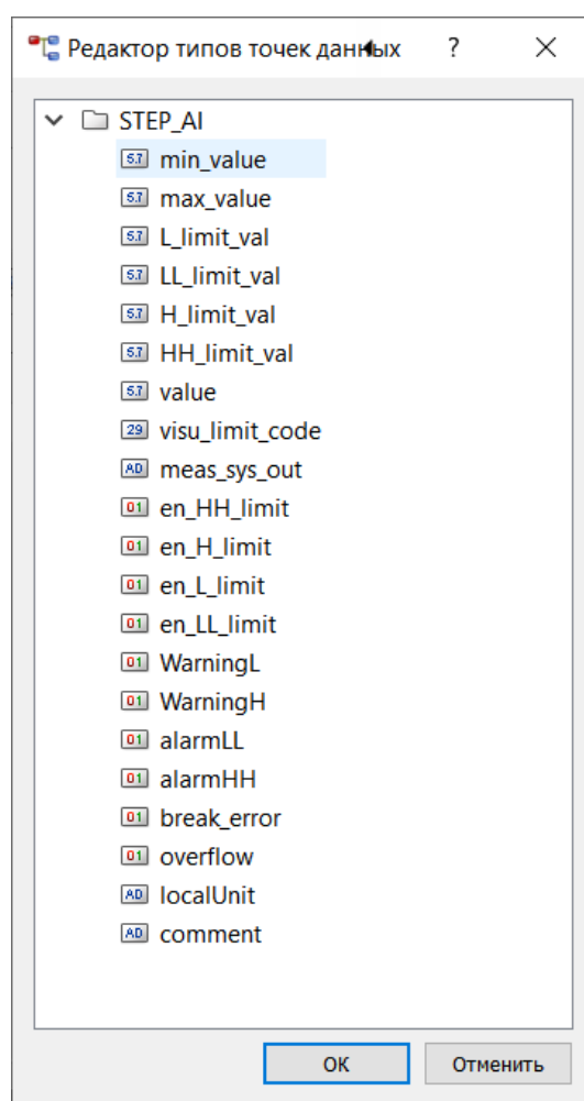
Рис. 7. Структура STEP_AI
