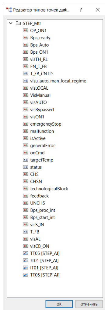
Рис. 8. Структура STEP_Mtr
