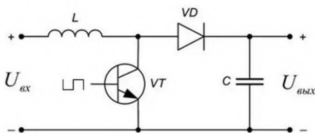
Рис. 1. Упрощенная электрическая схема повышающего преобразователя напряжения
