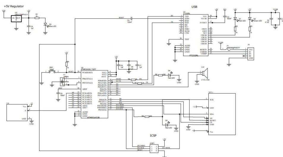
Рис. 3. Электрическая принципиальная схема устройства
