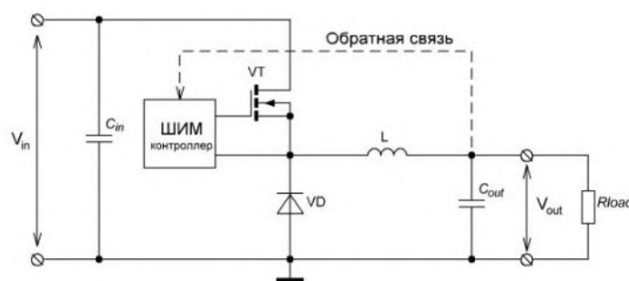
Рис. 2. Электрическая схема понижающего преобразователя постоянного напряжения
