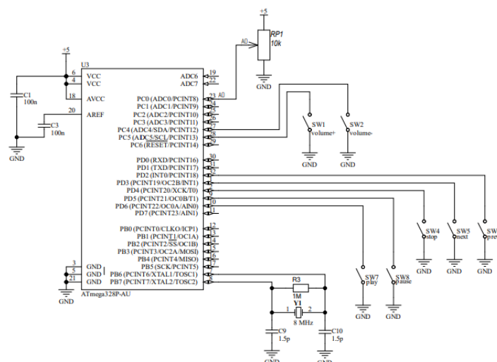
Рис. 2. Микроконтроллер ATmega328P на принципиальной электрической схеме
