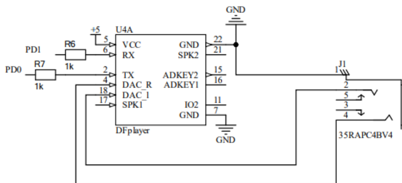
Рис. 3. Схема подключения аудиомодуля к микроконтроллеру в плеере
