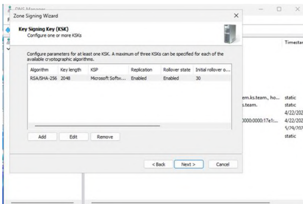
Рис. 2. Настройка DNSSec
