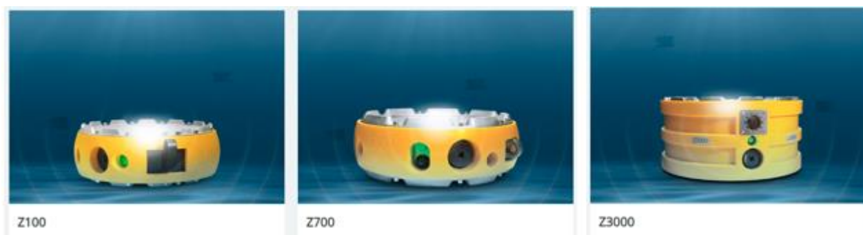
Рис. 2. Донные сейсмические станции Fairfield Nodal Z100, Z700 и Z3000
