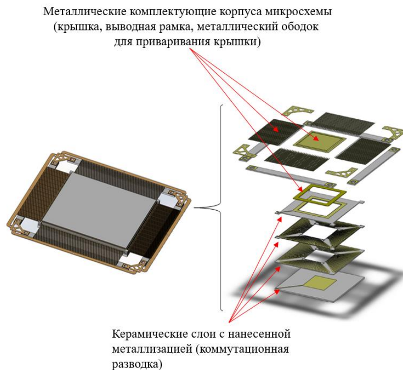
Рис. 1. Схематическая конструкция металлокерамического корпуса
