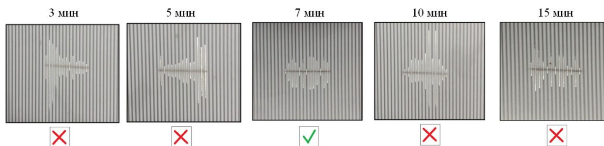
Рис. 7. Модель имитации распределения припоя ПСр-72 между металлизационными площадками корпуса, предназначенными для пайки выводной рамки
