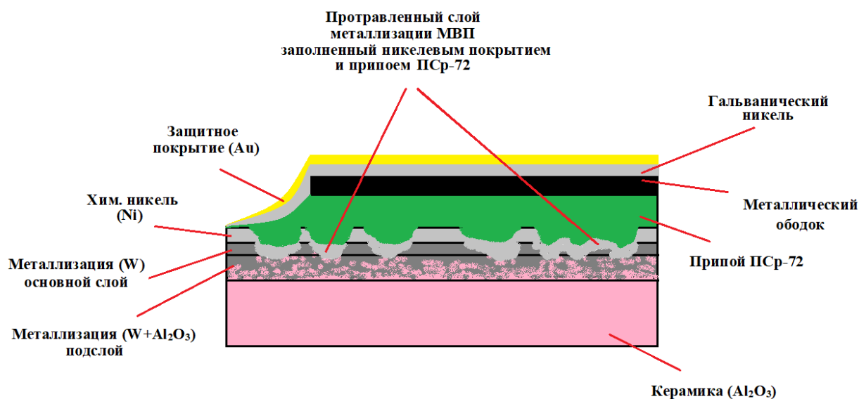
Рис. 6. Второй вариант металлокерамического соединения при наличии рыхлой поверхности металлизации
