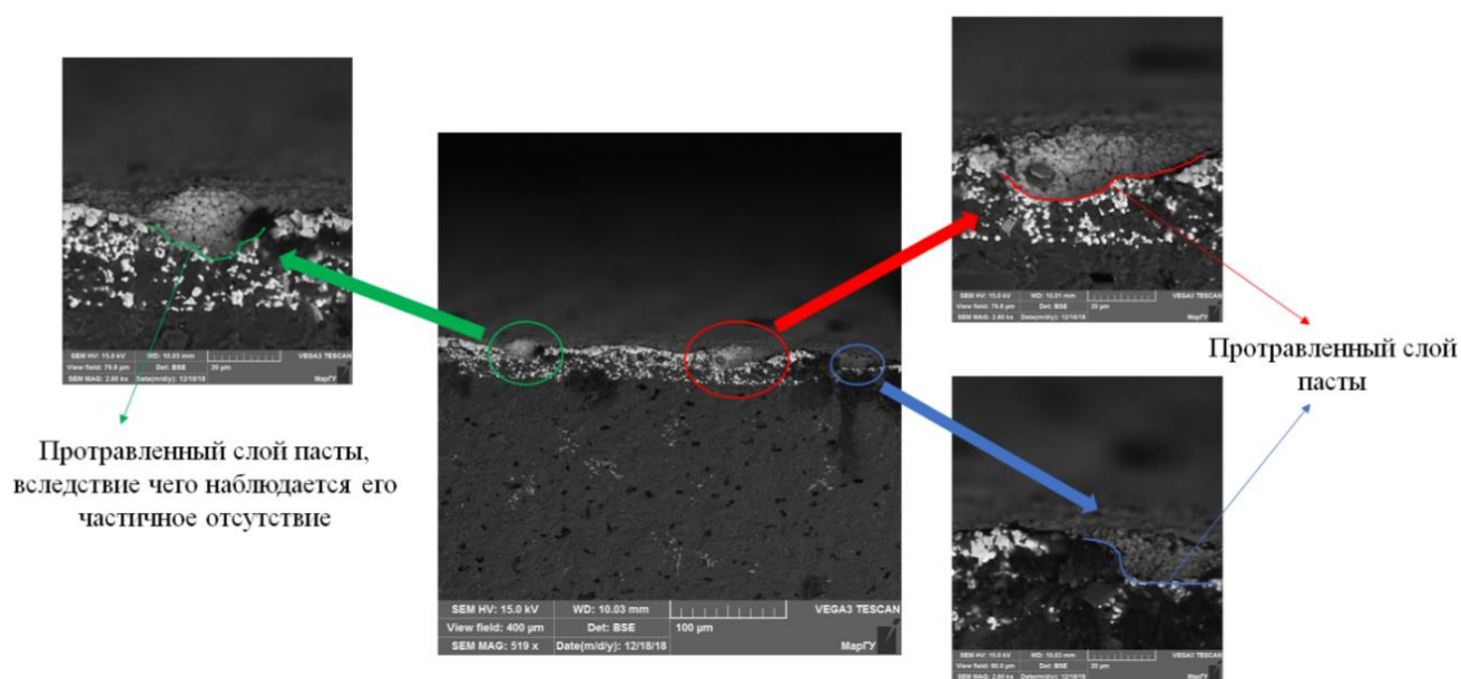
Рис. 4. Микроструктура поверхности металлизационного покрытия: время активации поверхности металлизации 15 минут, \times 2000
