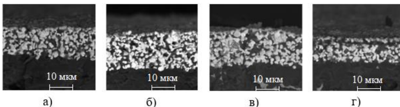
Рис. 3. Время активации поверхности металлизации в течение: а) 3 минуты, б) 5 минут, в) 10 минут, г) 15 минут
