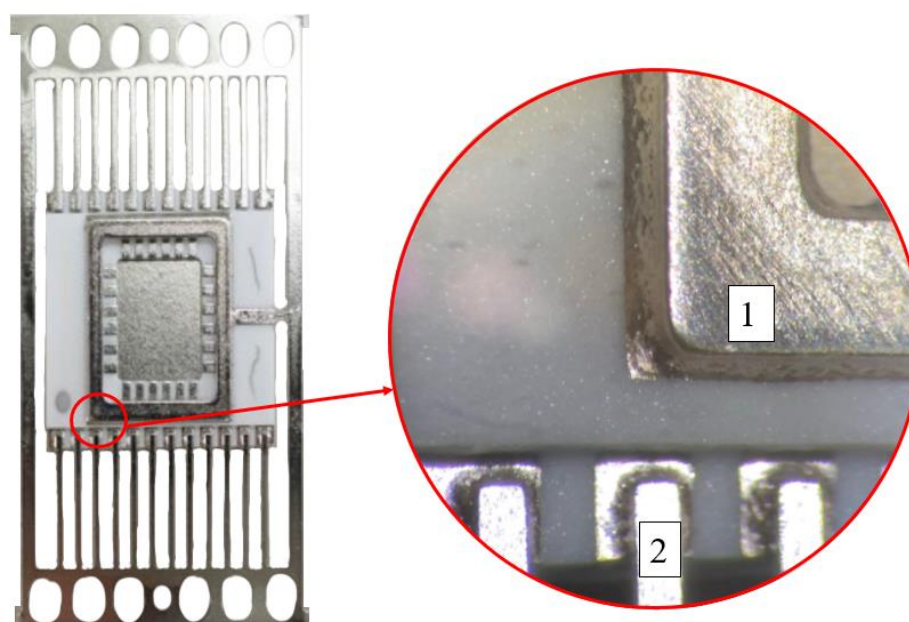
Рис. 2. Металлические навесные элементы корпуса микросхемы: 1 – металлический ободок; 2 – металлический вывод
