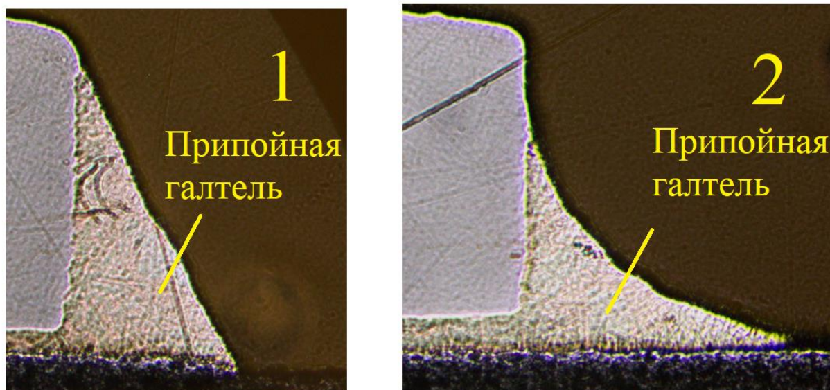
Рис. 9. Форма припойной галтели: 1 – время активации металлизации 15 минут; 2 – время активации 7 минут
