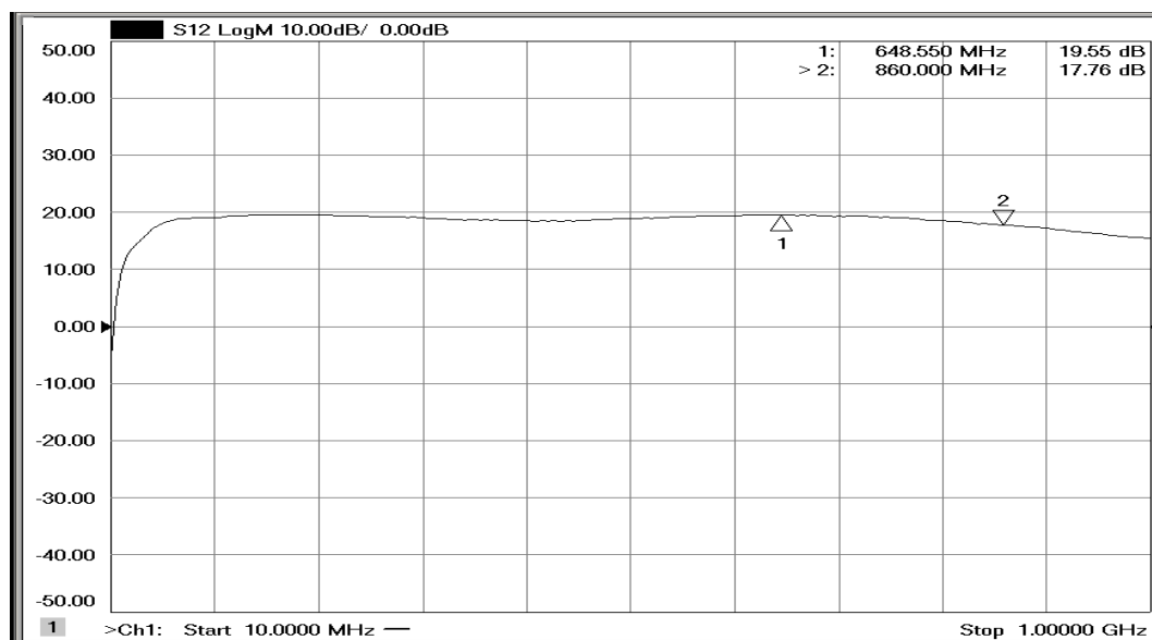
Рис. 4. АЧХ усилителя
