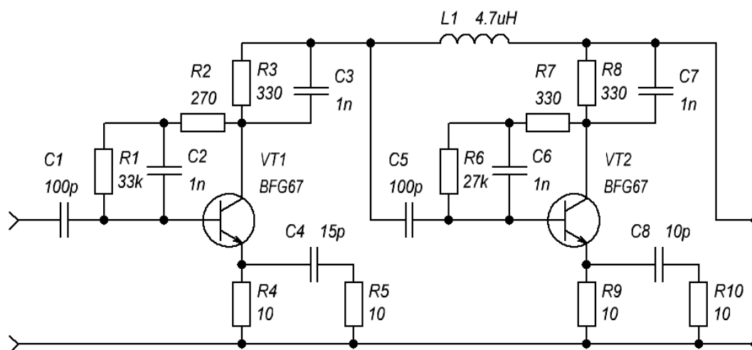
Рис. 1. Схема электрическая принципиальная [15]
