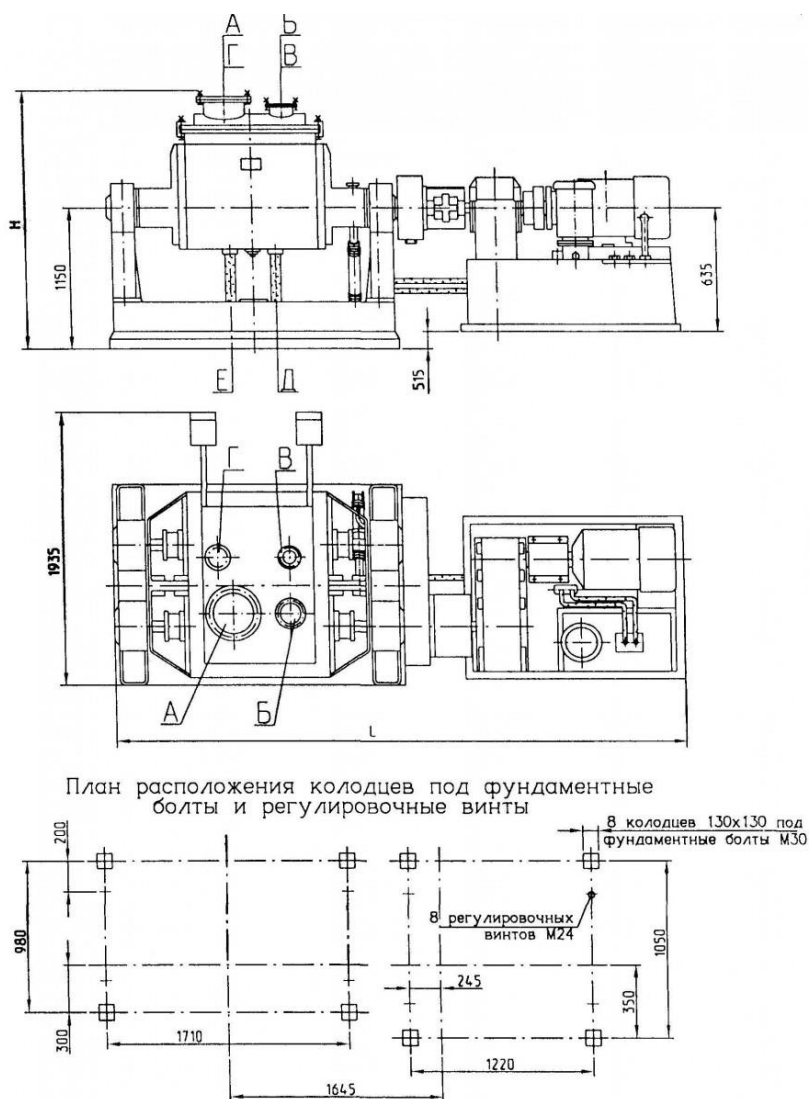
Рис. 1. Эскиз смесителя
