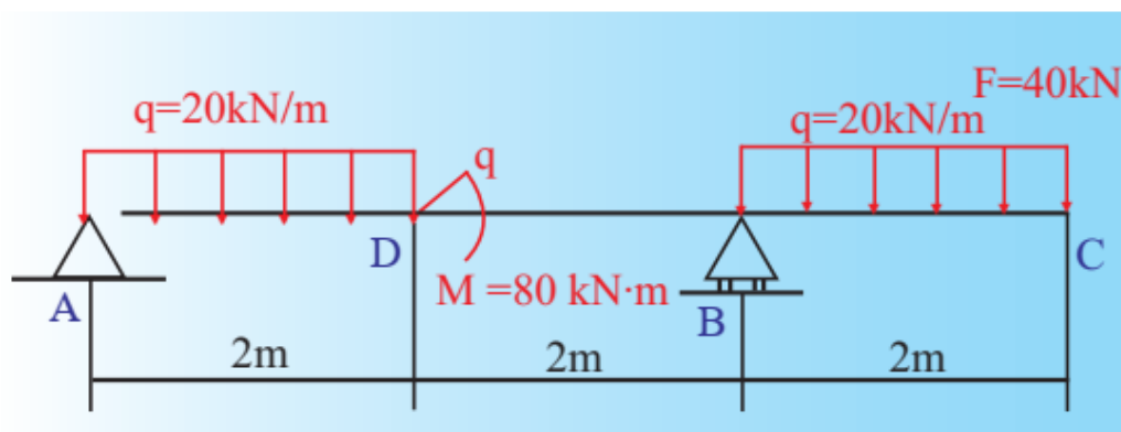
Рис. 3. Балка под воздействием сложной нагрузки
