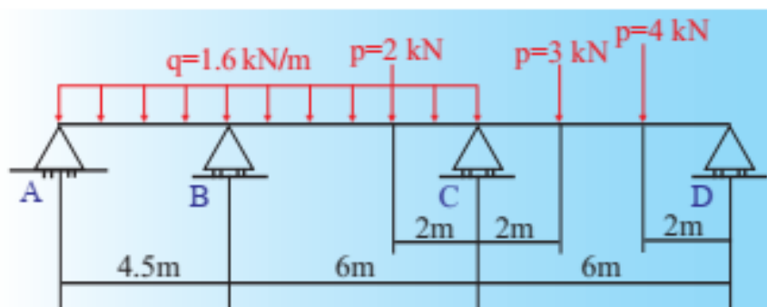
Рис. 6. Статически неопределимая балка, испытывающая сложную нагрузку
