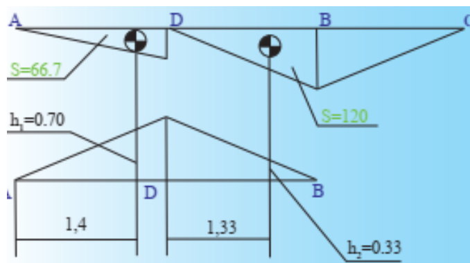
Рис. 4. Определение кривой в точке D с помощью программы AutoCAD
