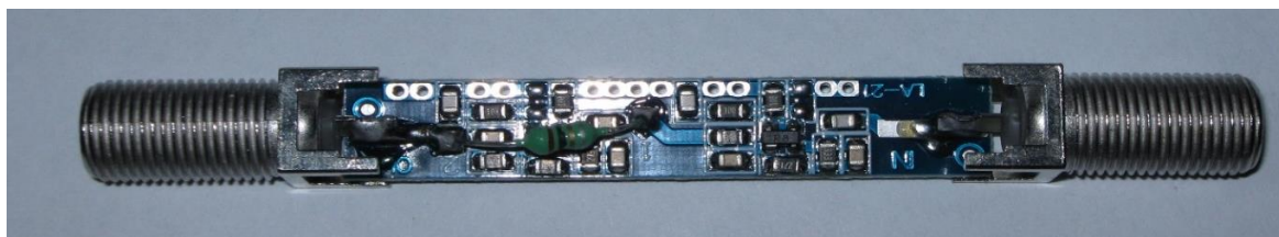
Рис. 2. Фото усилителя со снятым корпусом
