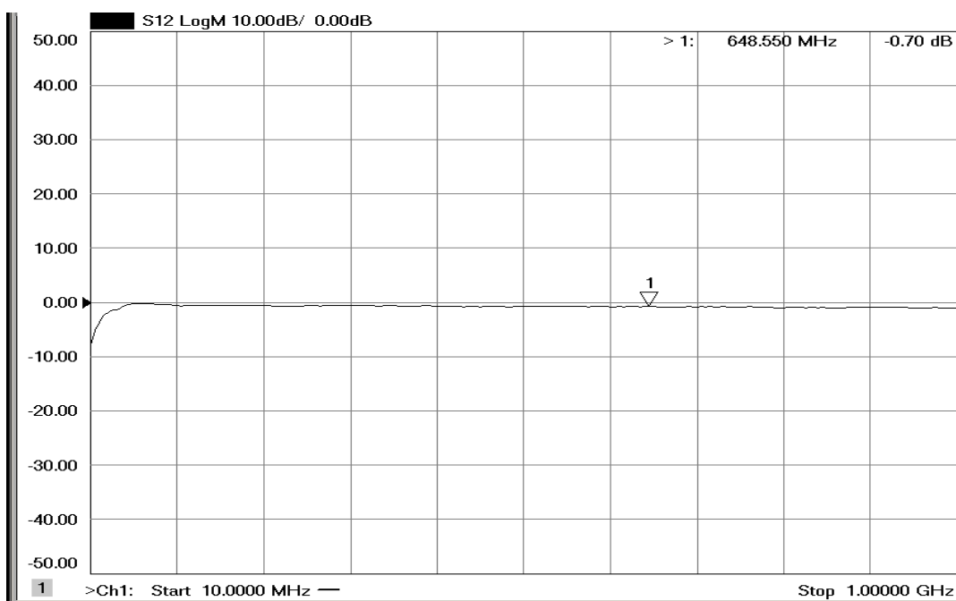
Рис. 5. Потери в устройстве подачи питания
