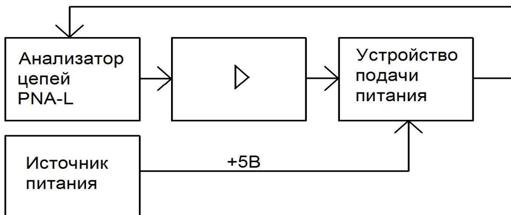
Рис. 3. Структурная схема измерительной установки
