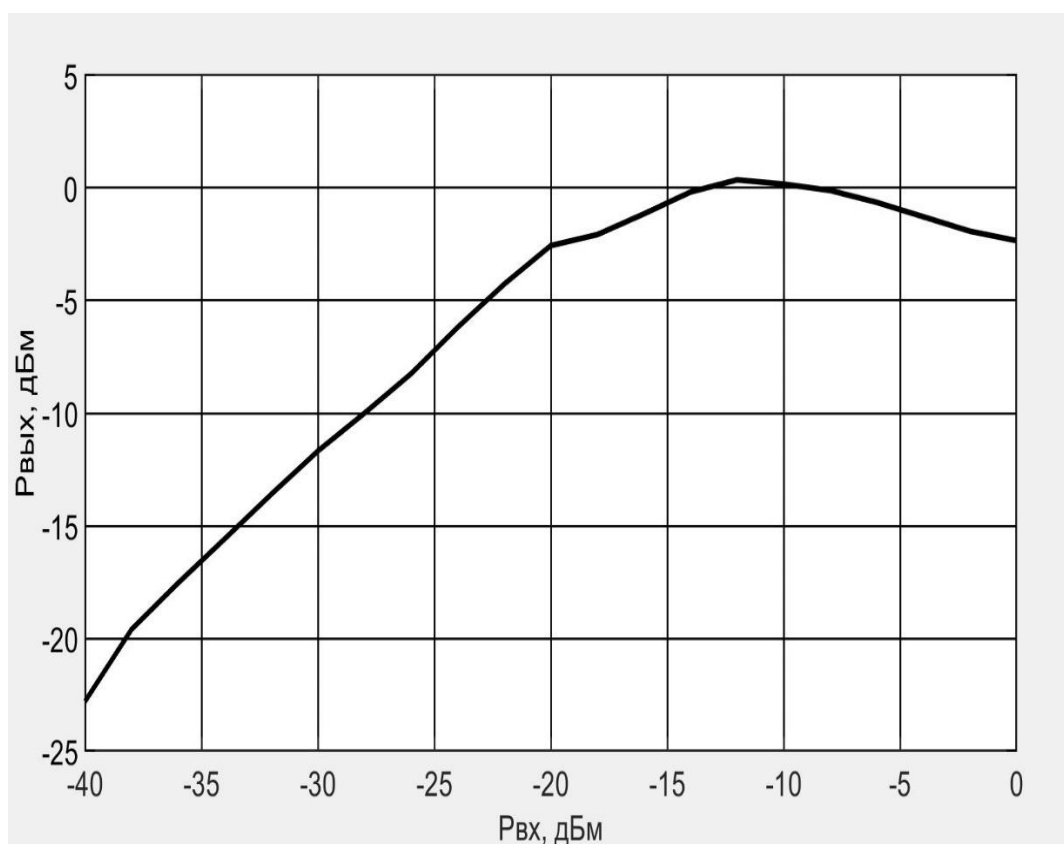
Рис. 6. Амплитудная характеристика на частоте 800 МГц
