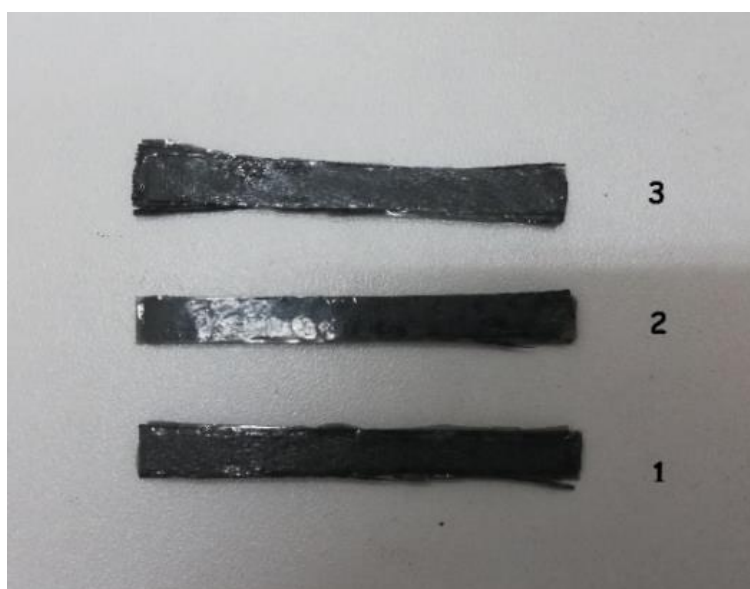
Рис. 3. Образцы многослойной структуры, созданные методом ультразвукового ламинирования
