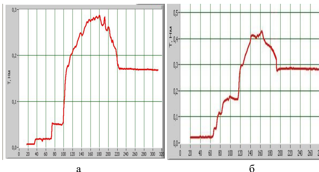
Рис. 6. Кинетика нагружения образца из ПКМ: 6 слоя УП препрега и 7 слоёв полимера (а); 10 слоёв УП препрега и 11 слоёв полимера (б)
