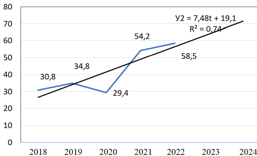
Рис. 3. Динамика количества калибровок и уравнение регрессии
