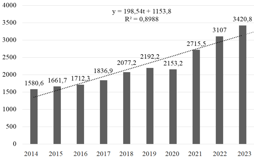
Рис. 1. Динамика и уравнение регрессии расходов на метрологию, млрд. руб.
