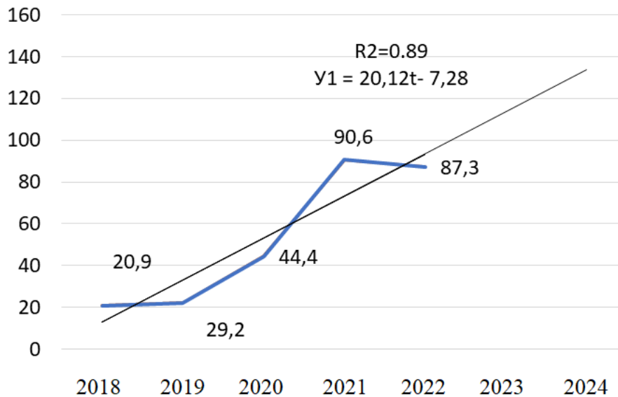
Рис. 2. Динамика количества проверок и уравнение регрессии
