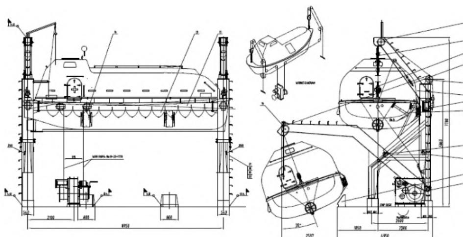
Рис. 4. Чертеж шлюпки закрытого типа
