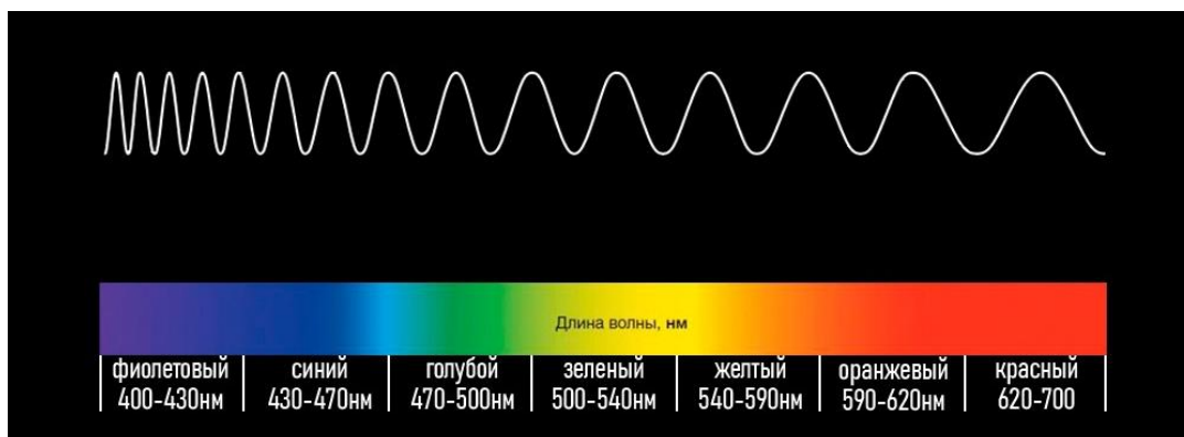
Рис. 2. Схема длины волн в физическом восприятии
